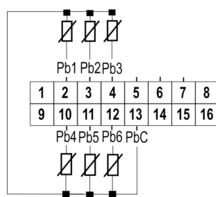
IPG-IPC 4 DIN
